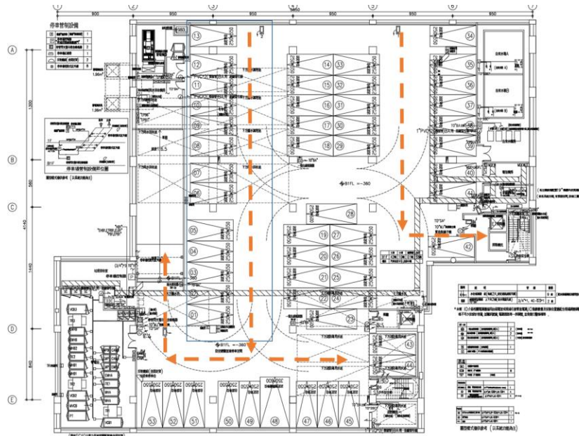
化工二館地下樓疏散路線圖
