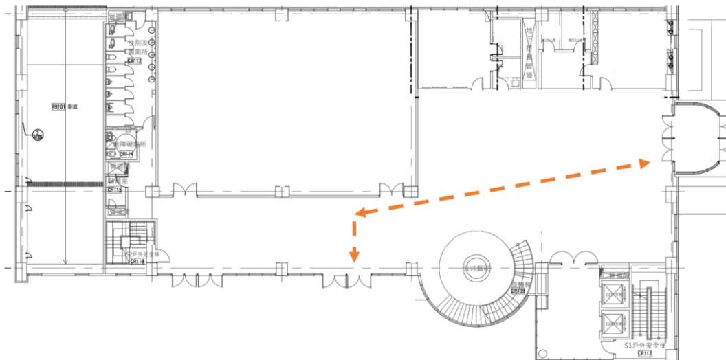
化工二館一樓疏散路線圖
